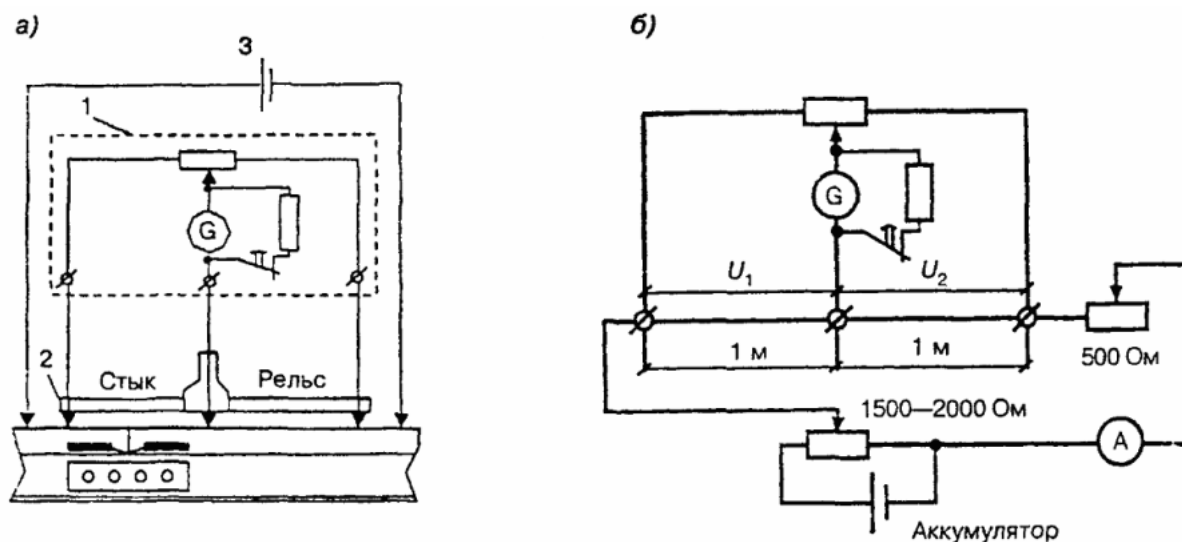
Рисунок 2. - Схемы измерения сопротивления сборного стыка ходового рельса (а) и проверки стыкоизмерителя (б)
