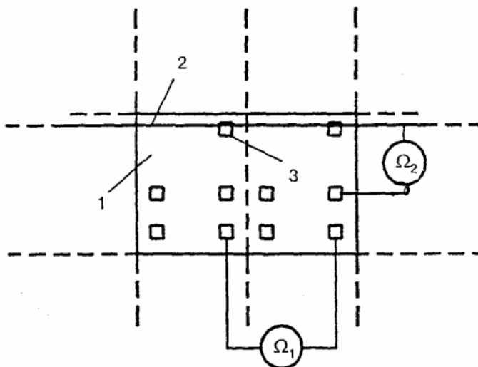
Рисунок 8. - Схема проверки наличия гальванической связи между арматурой железобетонных блоков ( \Omega_1 ), арматурой и шиной заземления ( \Omega_2 )
