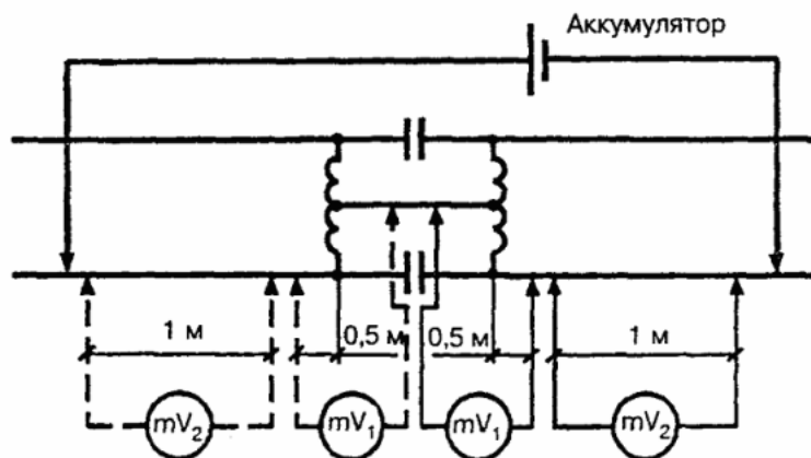
Рисунок 4. - Схема измерения сопротивления изолирующего стыка ходового рельса с ДТ
