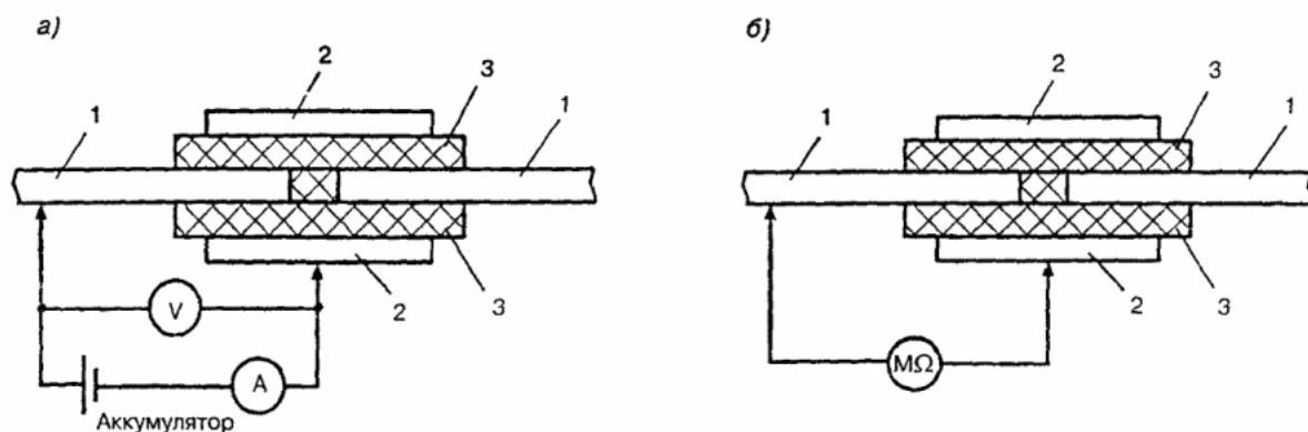
Рисунок 5. - Схема измерения сопротивления изоляции стыка ходового рельса
