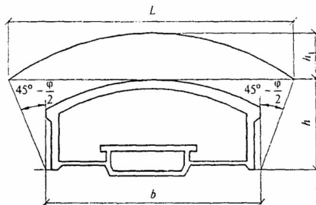
Рисунок 1. - Схема для расчета высоты свода обрушения
