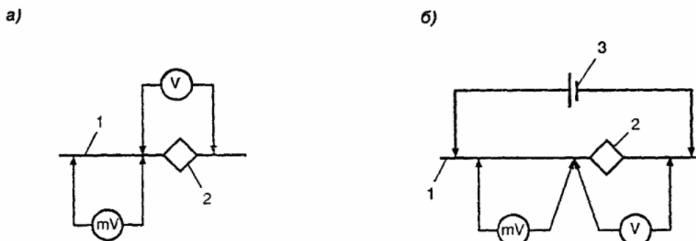
Рисунок 6. - Схема контроля состояния изолирующих муфт на кабелях приблизительно без источника тока (а) и с источником тока (б)
